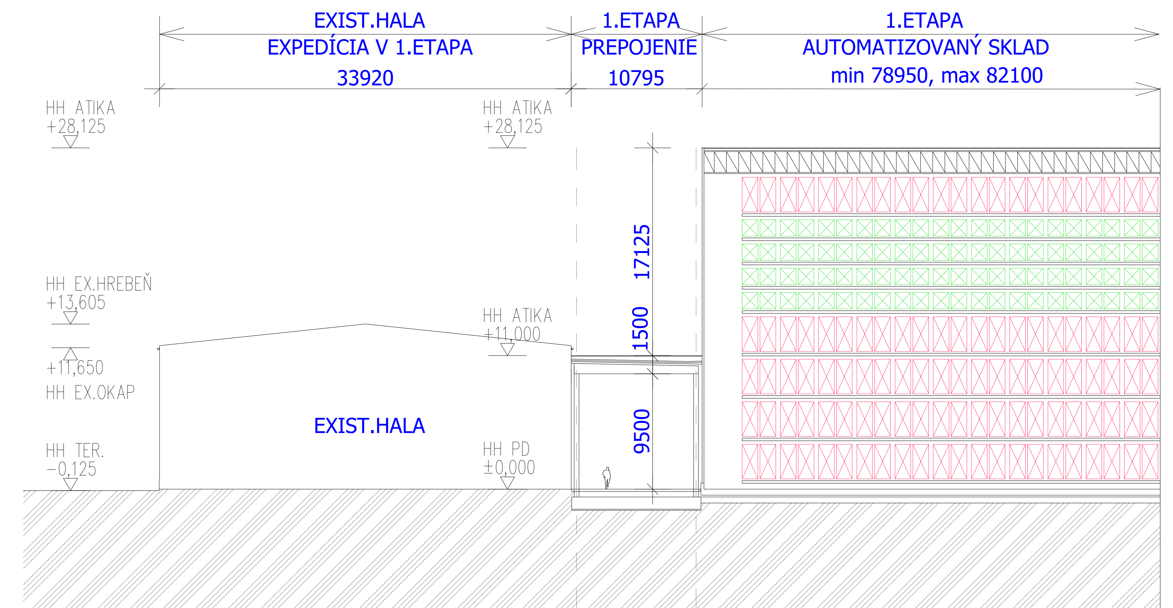
REZ B-B
