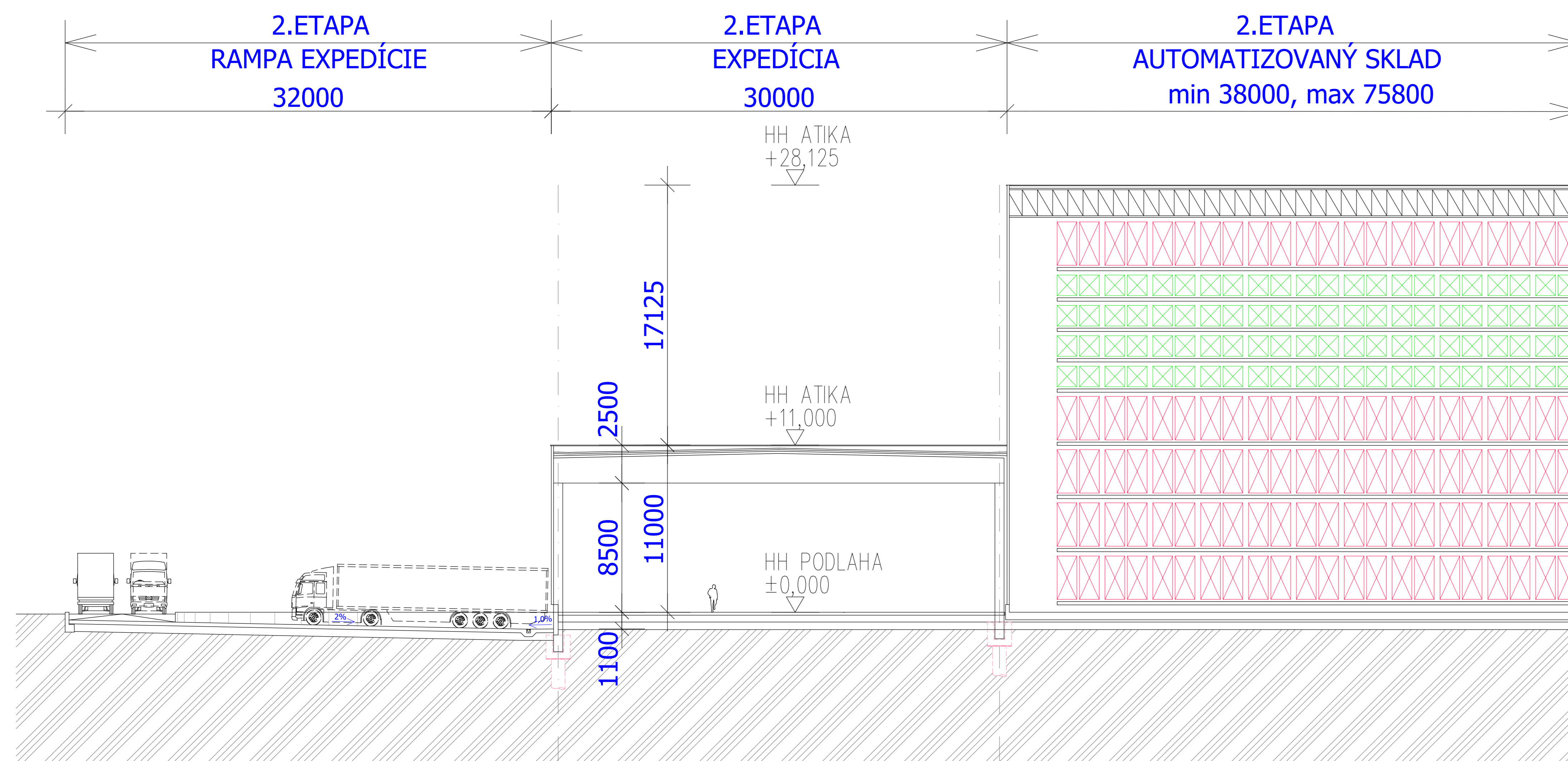
REZ C-C
